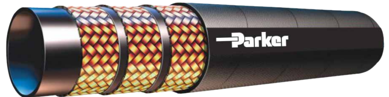
Tuyau de terrain tuyau de trou mince (3 fils)
